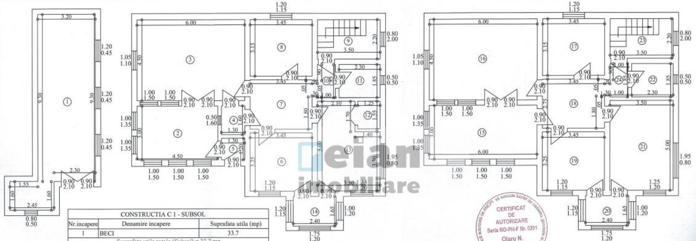
RELEVU CONSTRUCTIE C1 SUBSOL, SCARA 1 : 100
